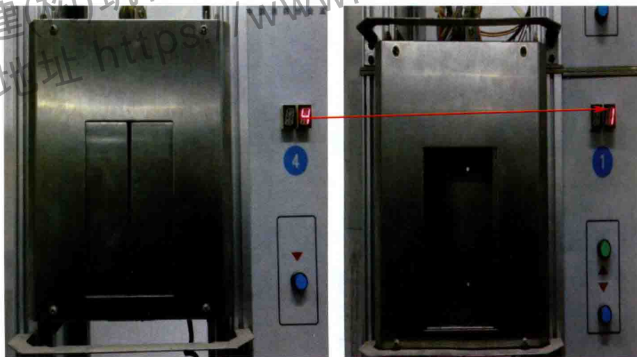
图 10-57 消防电梯迫降首层
