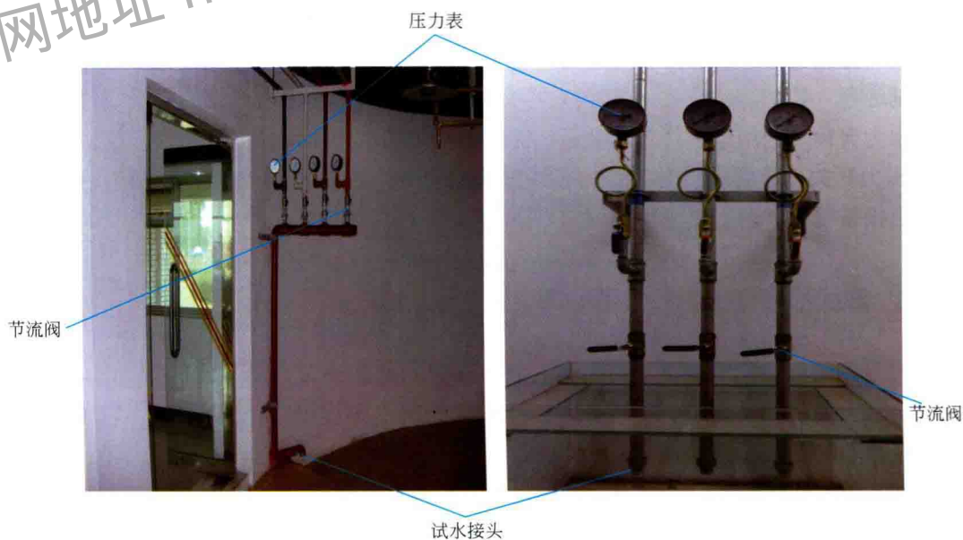
图 10-23 末端试水装置
