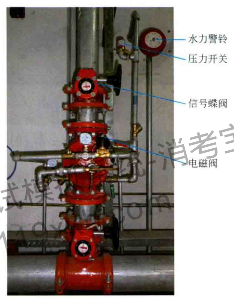
图 10-18 雨淋自动喷水灭火系统
